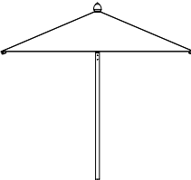
Ø 6 / Ø 350 H 277 - Ø 400 H 295
